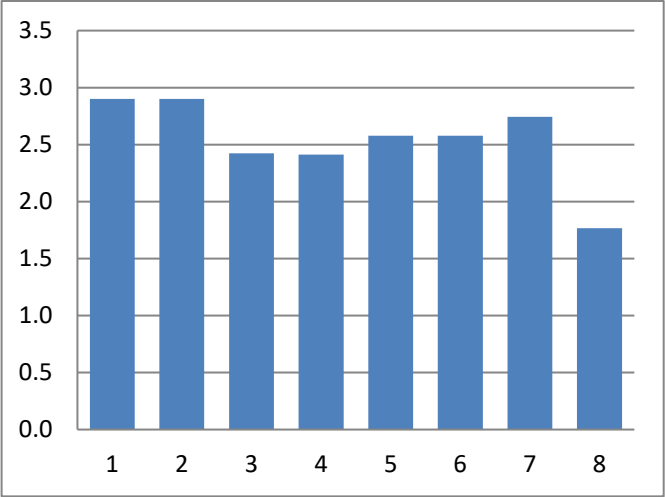
PO
