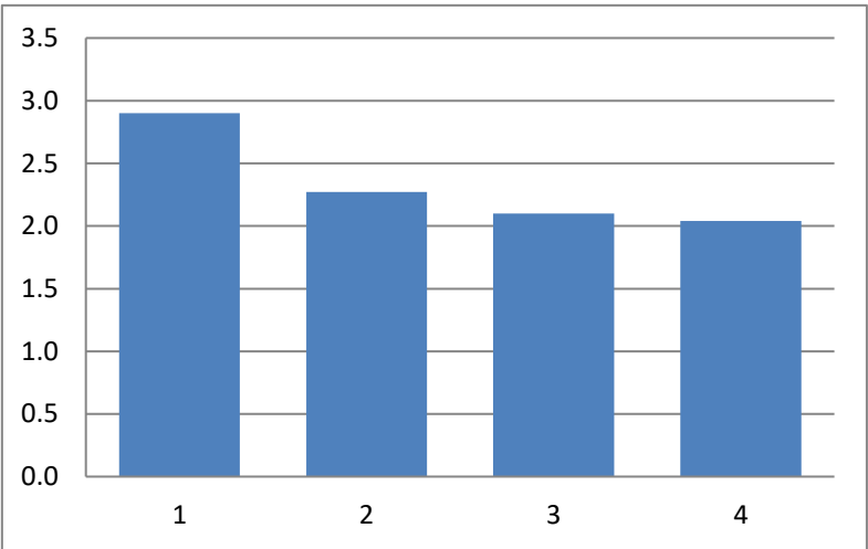
PSO
